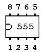
CIRCUITO INTEGRADO
